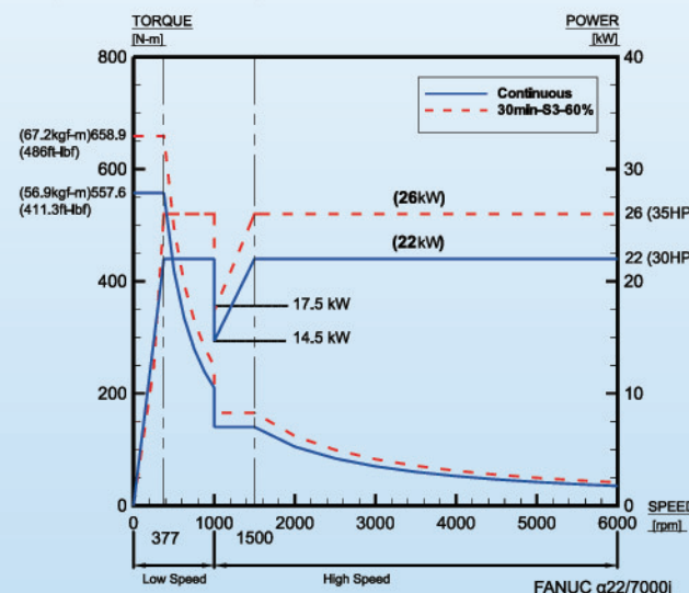
■ Gear type spindle, 22/26kW, 6000rpm (Standard: V22/32)
